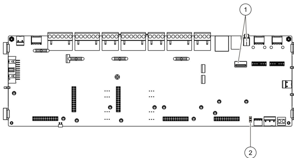
Figura 23: Conectores USB e JP4 na PCB do painel de controlo
