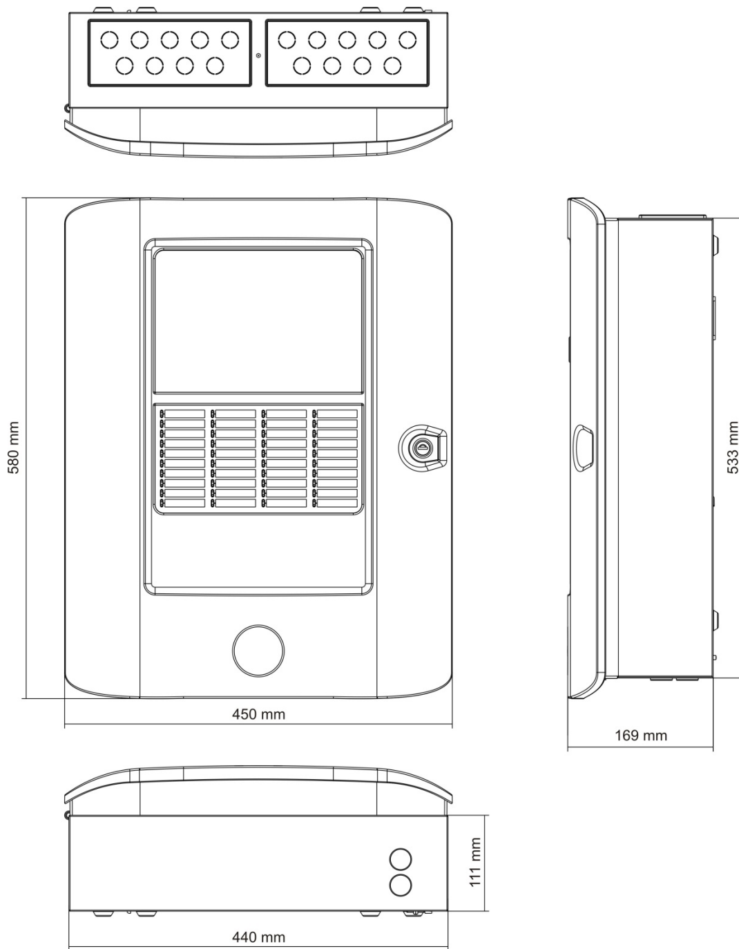
Figura 27: Dimensões e vistas da caixa grande
