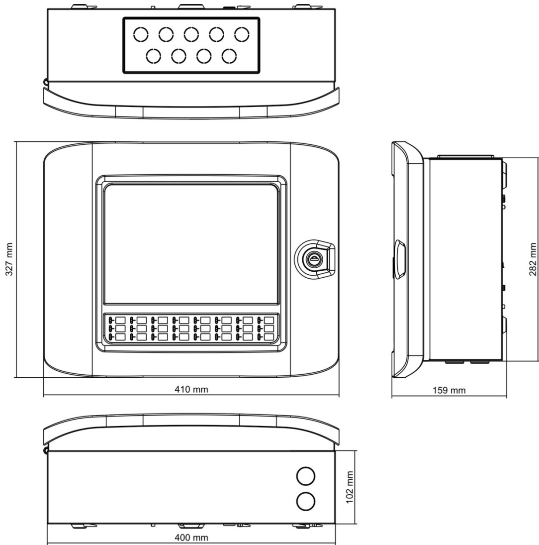
Figura 28: Dimensões e vistas da caixa pequena
