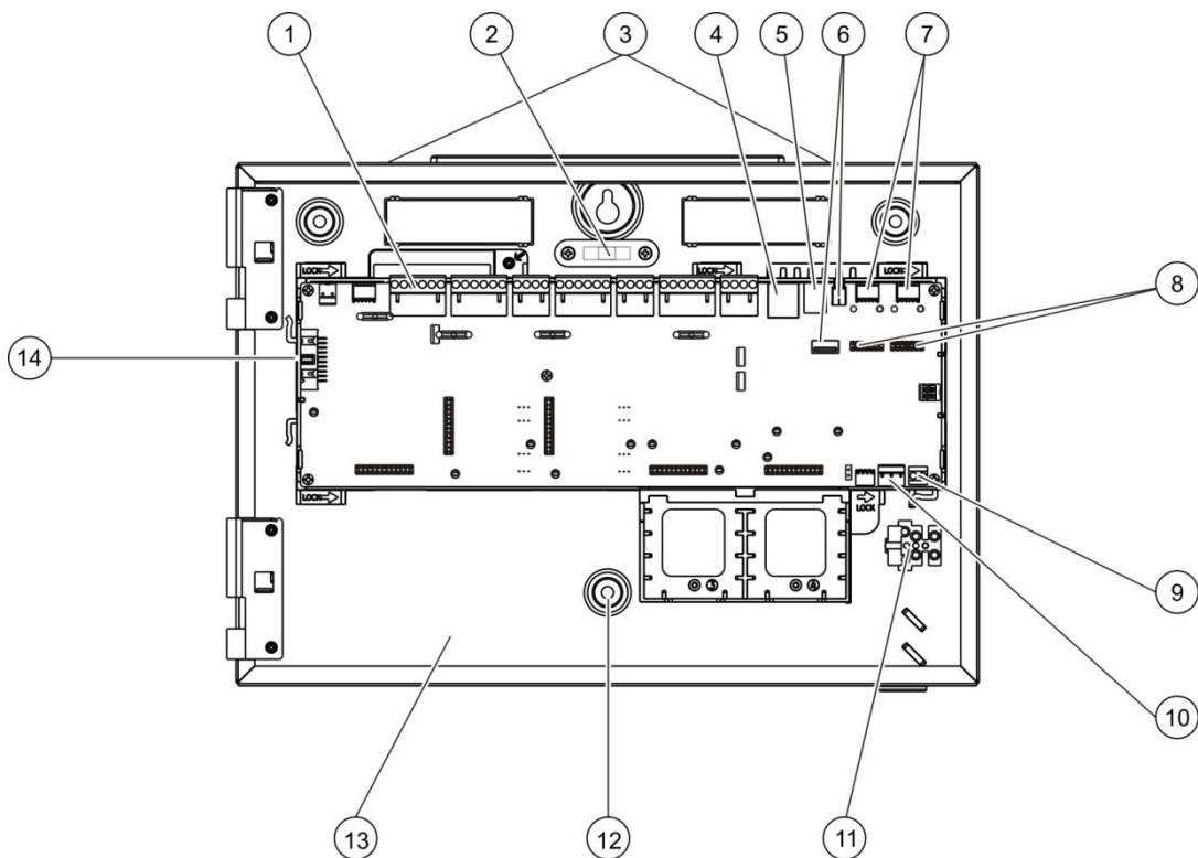
Figura 5: Esquema da caixa pequena e da PCB (Placa de circuito impresso) (painel de controlo de dois loops)
