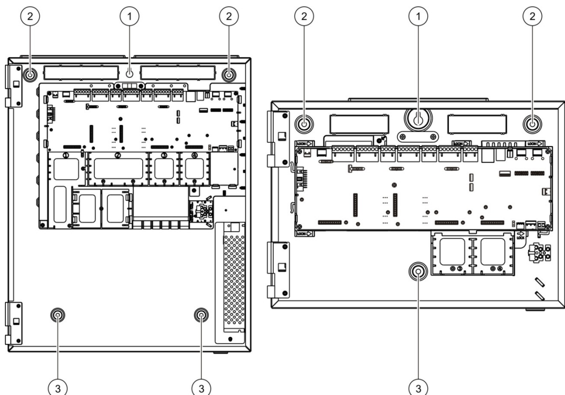
Figura 7: Localização dos orifícios de montagem
