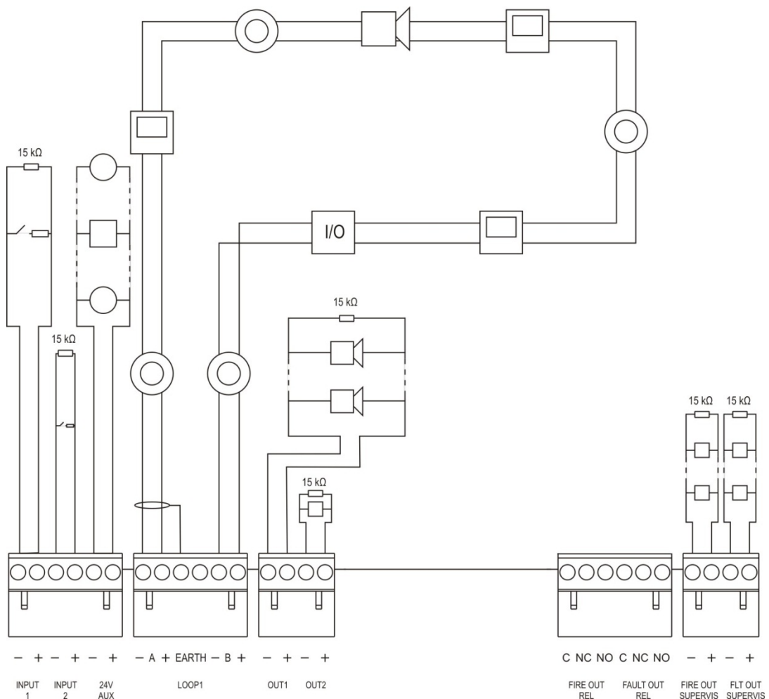
Figura 12: Descrição geral das ligações habituais do sistema de incêndio com um único loop de Classe A
