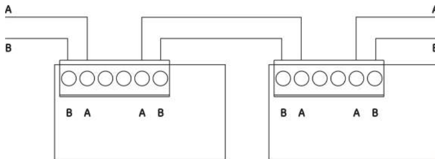
Figura 17: Ligações da placa de rede
