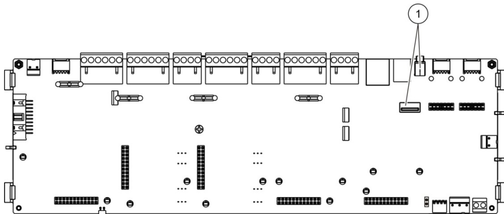
Figura 21: Conectores USB na PCB do painel de controlo
