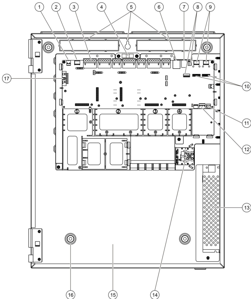
Figura 4: Esquema da caixa grande e da PCB (Placa de circuito impresso) (painel de controlo de dois loops)
