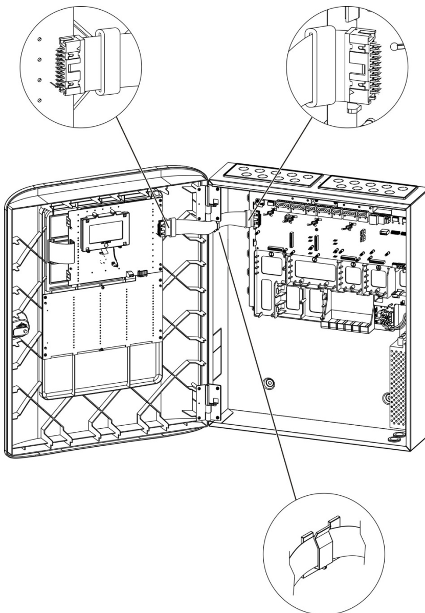
Figura 9: Ligar o cabo de interface do utilizador
