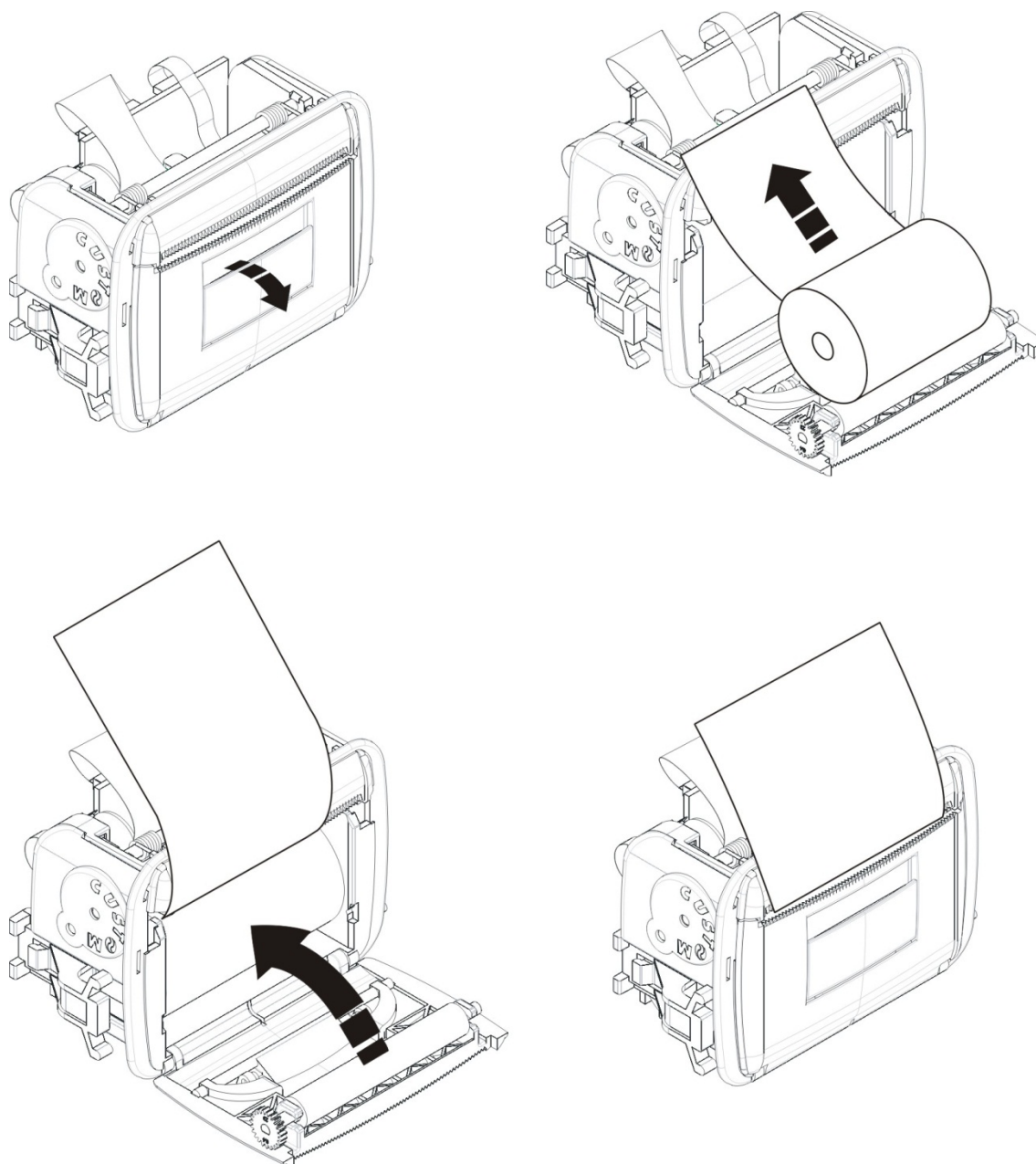
Figura 11: Colocar o papel na impressora interna
