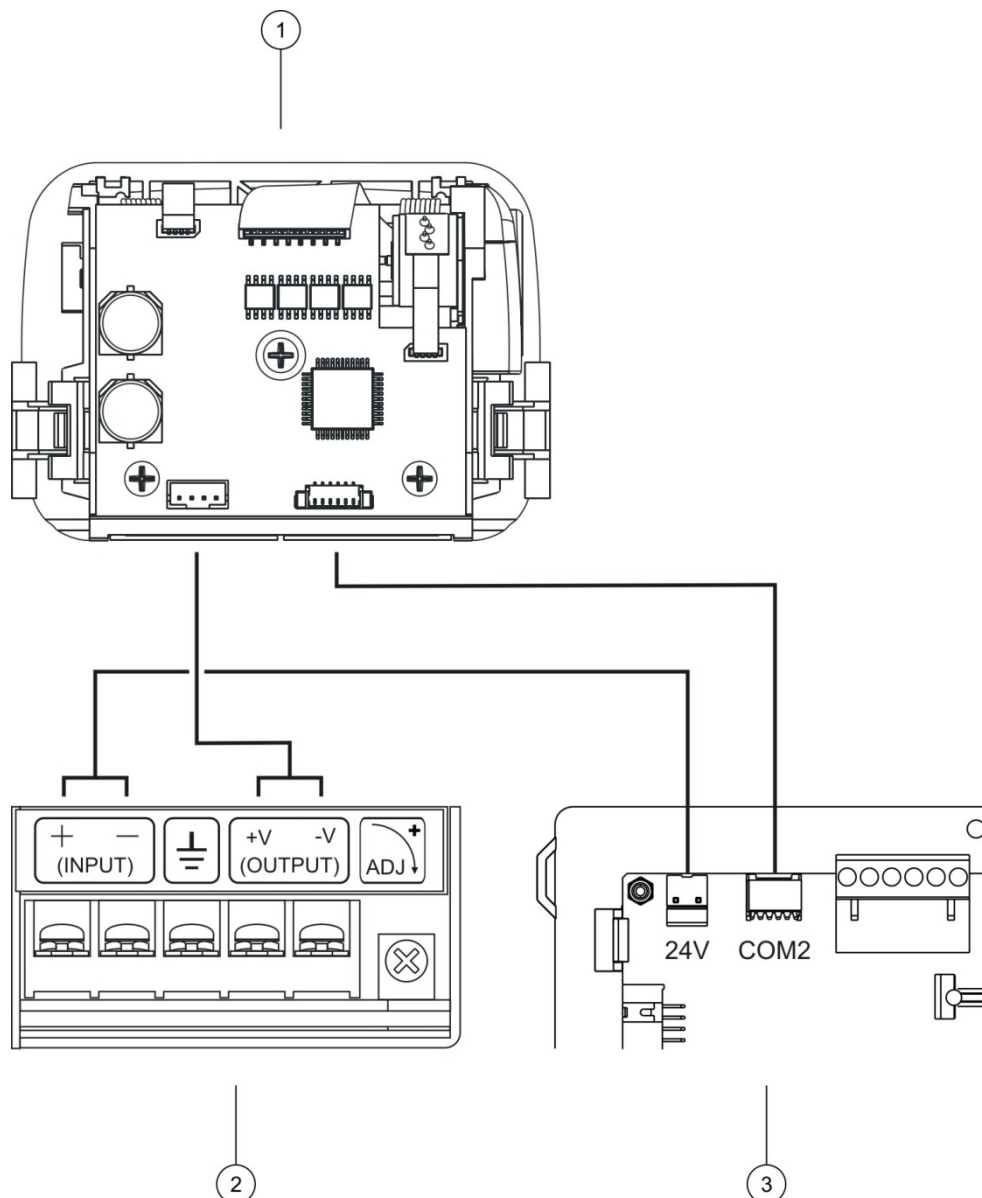
Figura 10: Ligar a impressora interna
