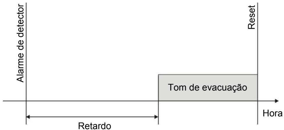
Figura 25: Alarme de detector com retardo standard (sem segunda fase)
