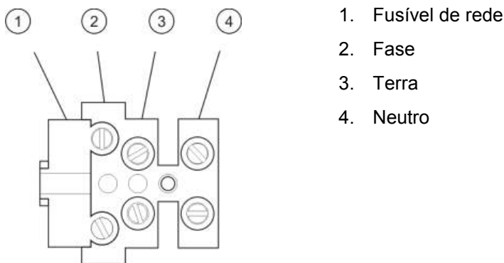
Figura 15: Ligação da alimentação de rede
