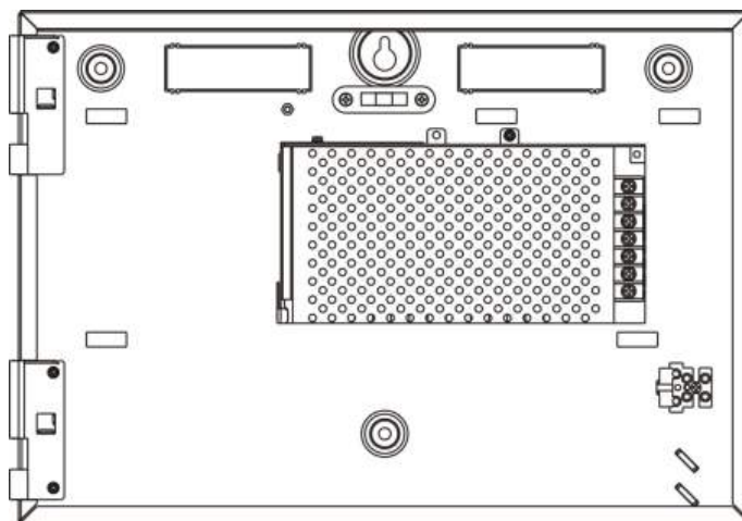
Figura 6: Caixa pequena, com a PCB principal e o chassis removidos, mostrando a fonte de alimentação
