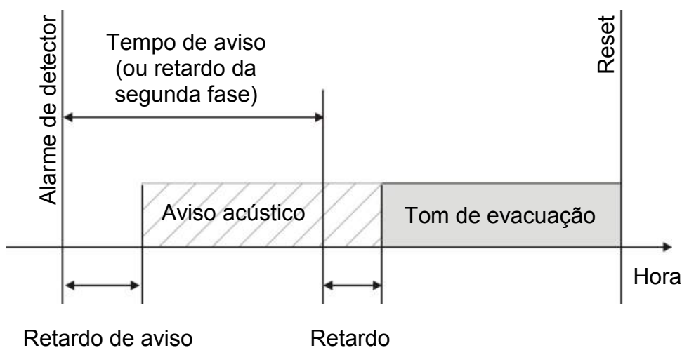
Figura 24: Alarme de detector com retardo da segunda fase
