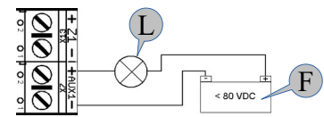
Figura 6: Exemplo de utilização das saídas auxiliares com uma lâmpada e bateria externa.
