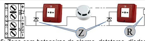
Figura 5: Zona com botoneiras de alarme, detetores, diodos zener e resistência de terminação.
